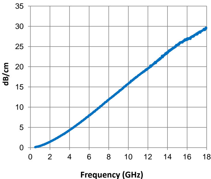
Attenuation
