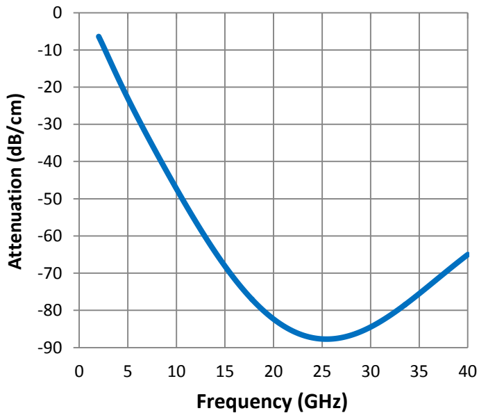
Attenuation
