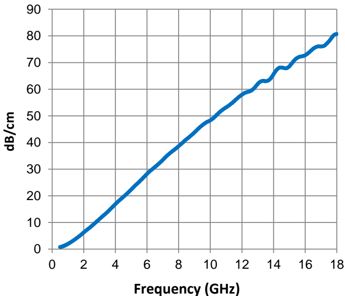
Attenuation
