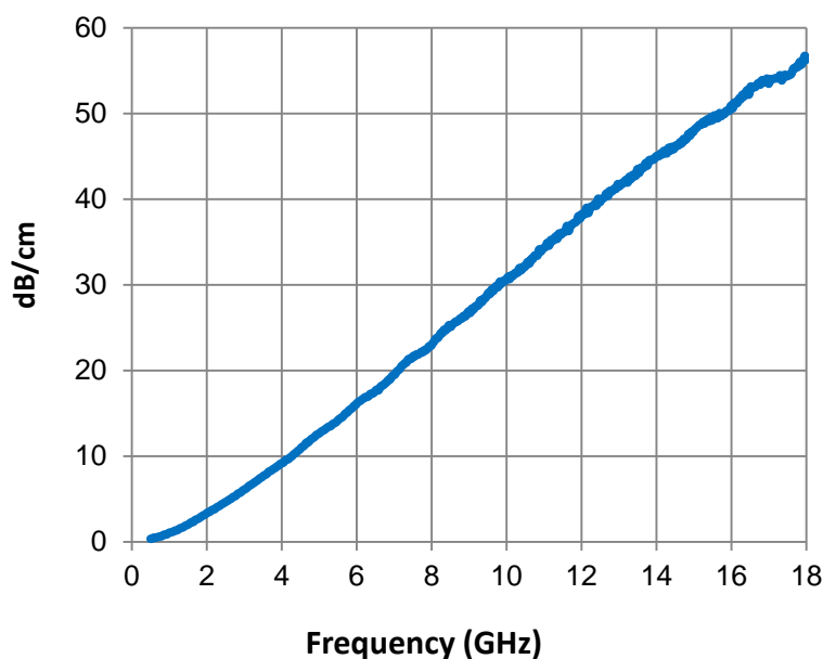
Attenuation
