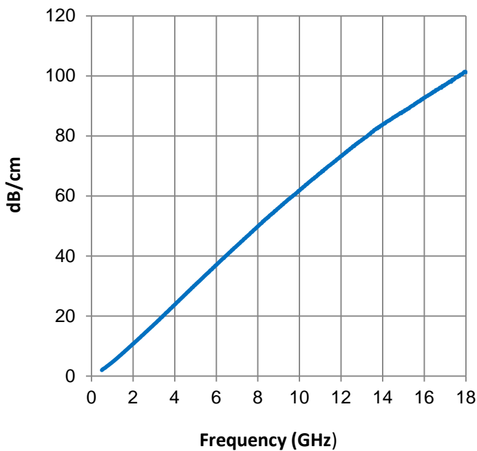
Attenuation
