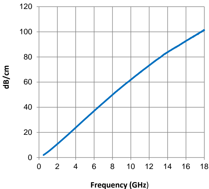
Attenuation
